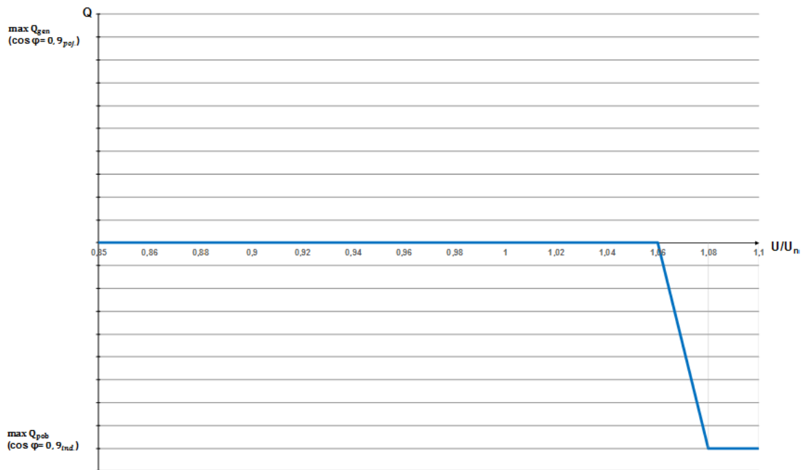
Rysunek 3 Charakterystyka sterowania mocą bierną w funkcji napięcia dla falowników podłączonych jednofazowo, wymagana przez OSDn
