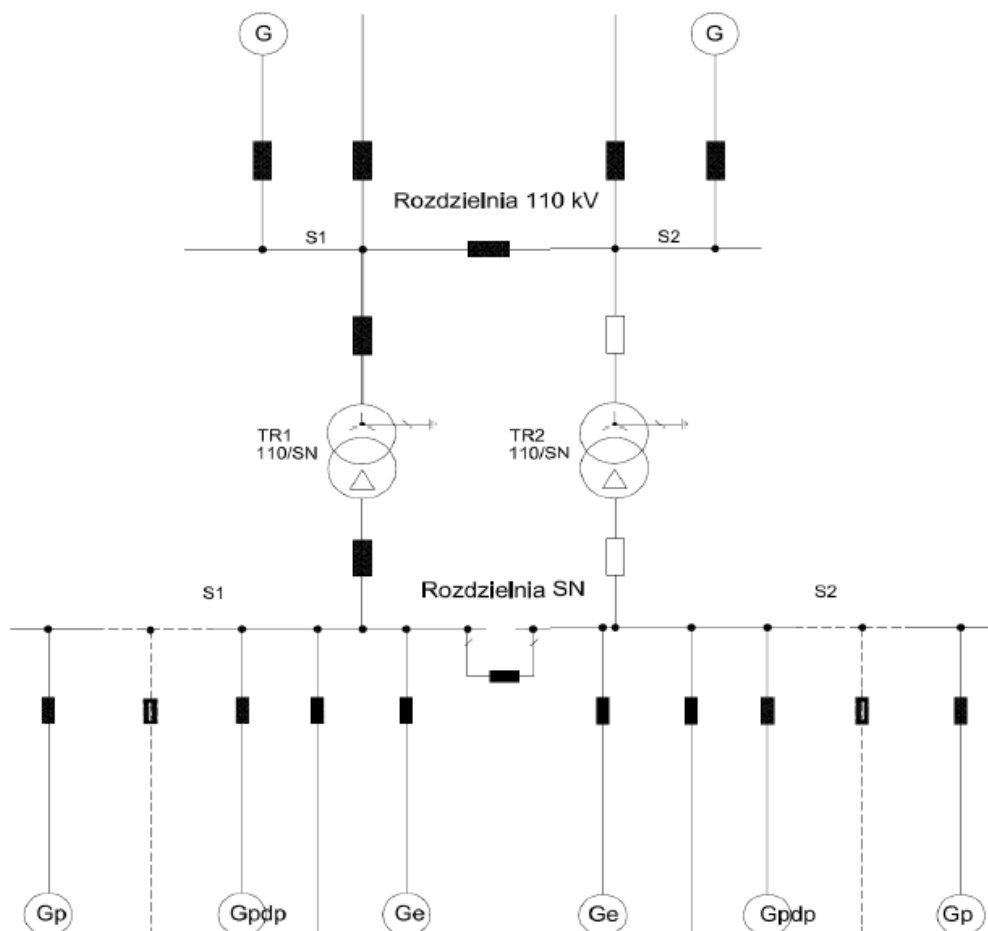
Rysunek 1 Konfiguracja maksymalna GPZ/RPZ
