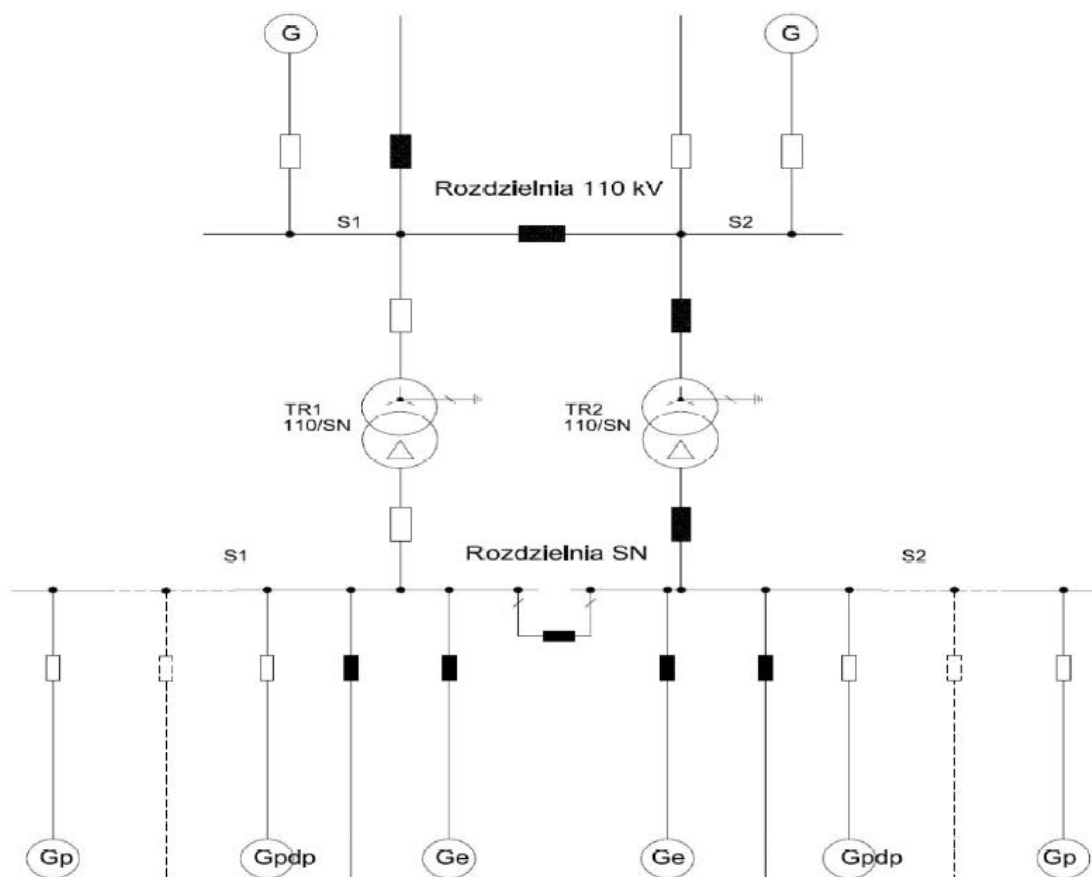
Rysunek 2 Konfiguracja minimalna GPZ/RPZ
